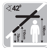
Finestra con asse di rotazione decentrato ed anta sottoluce
